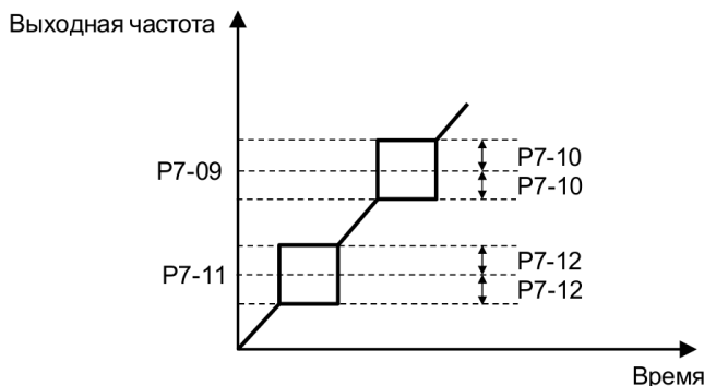
Рисунок 6.14 – Принцип работы функции скачкообразной перестройки
