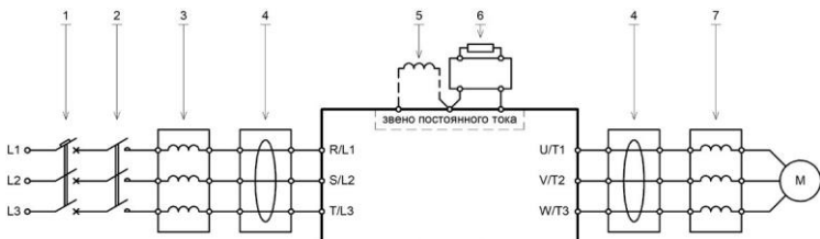
Рисунок 3.6 – Схема подключения дополнительного оборудования
