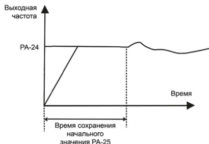
Рисунок 6.22 – Время сохранения опорного значения
