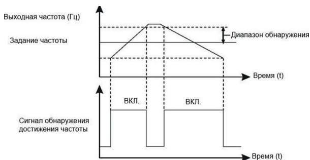
Рисунок 6.17 – Диапазон достижения максимальной частоты
