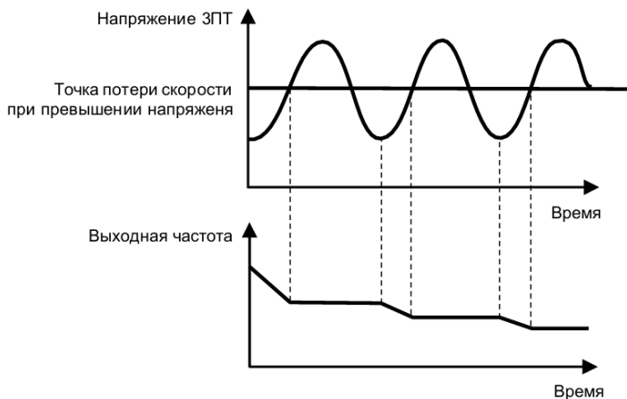
Рисунок 6.19 – Иллюстрация работы защиты от перенапряжения
