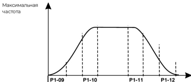
Рисунок 6.4 – S-образная кривая ускорения и замедления
