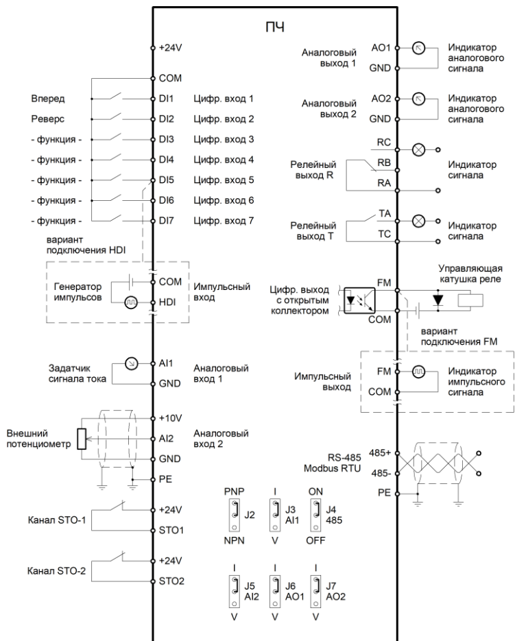
Рисунок 3.8 – Схема подключения управляющих клемм серии INPRIME MX
