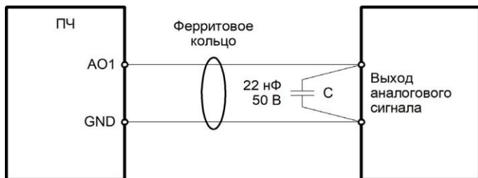
Рисунок 3.20 - Схема подключения проводов к аналоговому выходу (при воздействии сильных помех)
