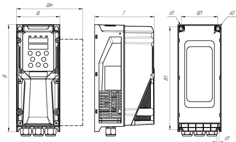
Рисунок 2.8а – Серия INPRIME MX IP65 в пластмассовом корпусе (типоразмеры 1-3)
