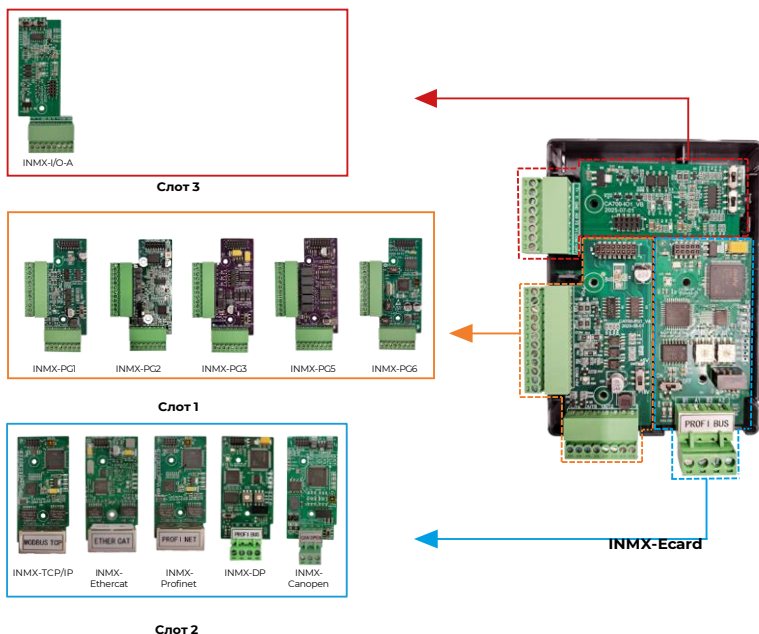
Рисунок 9.1 – Установка плат в модуль INMX-Ecard
