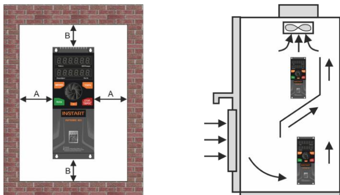
Рисунок 3.1 – Схема установки ПЧ серии INPRIME MX
