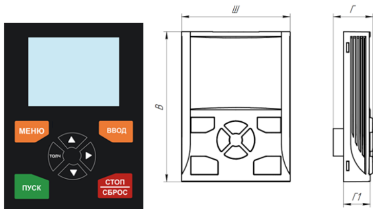
Рисунок 5.3 – Панель управления INPMX-KP-LCD
