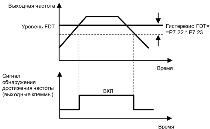
Рисунок 6.16 – Значение обнаружения выходной частоты
