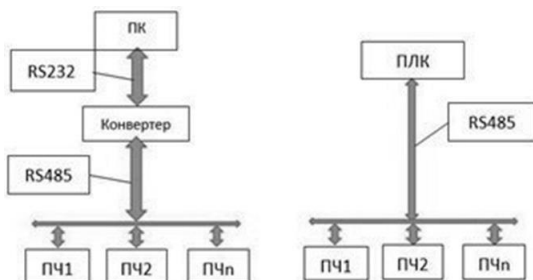
Рисунок 7.2 – Сетевой режим Master/Slaves
