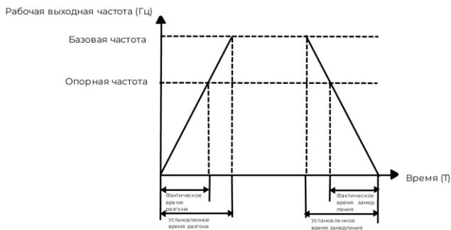
Рисунок 6.3 – Время разгона/замедления
