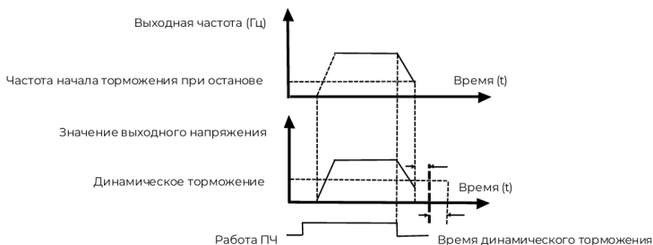
Рисунок 6.5 – Процесс торможения постоянным током
