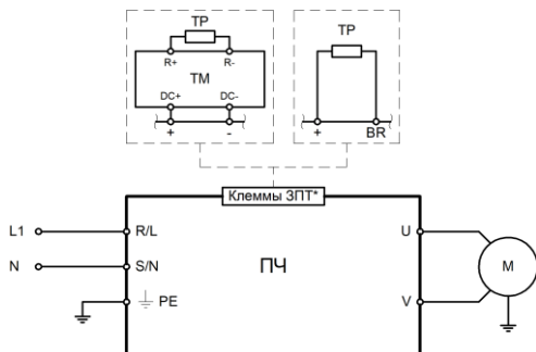
Рисунок 3.2 – Схема силовых подключений для моделей INPRIME MX- GY-1B
