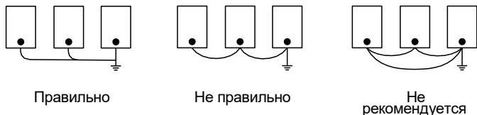
Рисунок 3.9 – Схематичное изображение образования петли с заземляющим проводом
