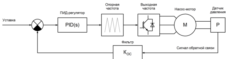
Рисунок 6.20 – Схема ПИД-регулирования
