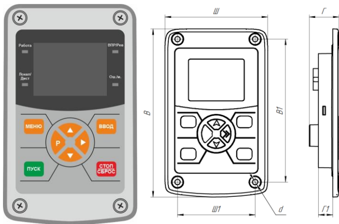
Рисунок 5.5 – Панель управления INPMX-KP-LCD IP65
