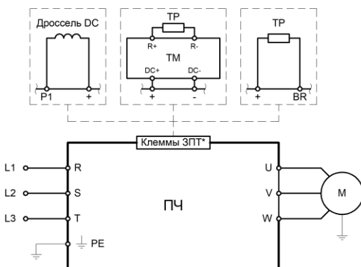
Рисунок 3.4 – Схема силовых подключений для моделей INPRIME MX- GY-3B
