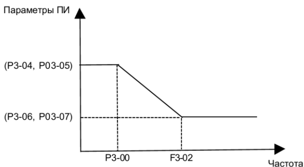
Рисунок 6.8 – Зависимость параметров ПИ от частоты
