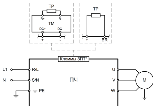
Рисунок 3.3 – Схема силовых подключений для моделей INPRIME MX- GY-2B
