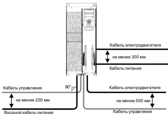
Рисунок 3.11 – Графическое представление расстояний между кабелями
