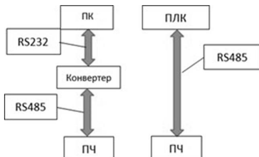
Рис. 7.1 Сетевой режим Master/Slave
