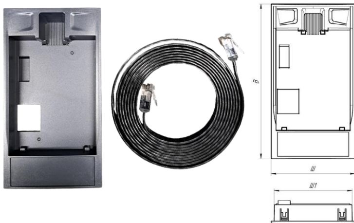
Рисунок 5.6 – Монтажный комплект INMX-MK и чертеж монтажной рамки INMX-MF
