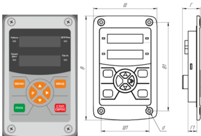
Рисунок 5.4 – Панель управления INPMX-KP-LED IP65
