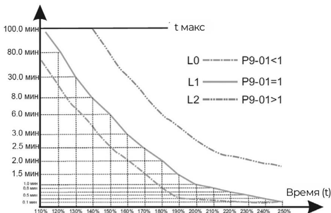
Рисунок 6.18 – Обратнозависимая времятоковая характеристика
