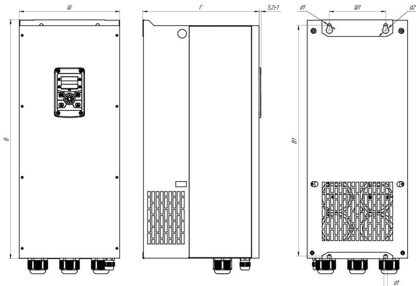
Рисунок 2.8а – Серия INPRIME MX IP65 в пластмассовом корпусе (типоразмеры 4-12)
