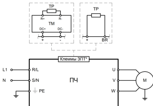
Рисунок 3.4 – Схема силовых подключений для моделей INPRIME MX- GY-3B
