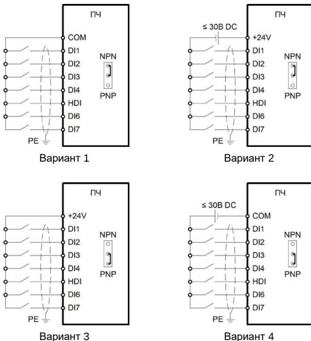
Рисунок 3.15 – Варианты подключения цифровых клемм
